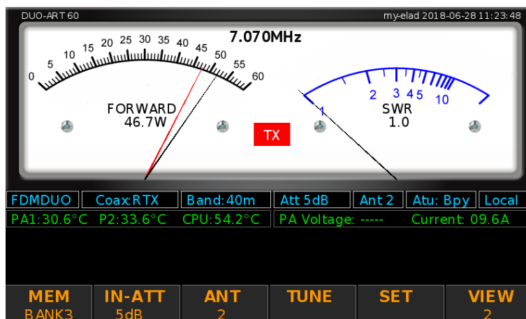
VIEW 2 : potenza diretta e ROS (SWR).
